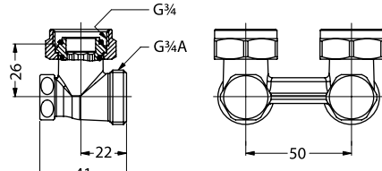
RLV-KS кутовий 003L0223
