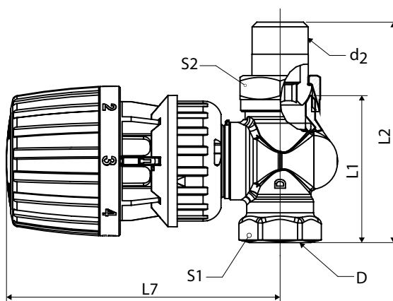
Прямий клапан RA-DV з термостатичним елементом RA 2991
