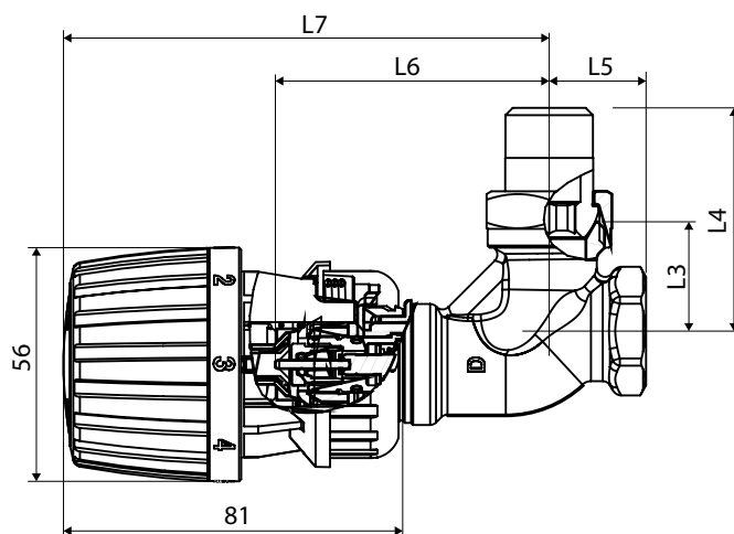
Кутовий клапан RA-DV з термостатичним елементом RA 2991
