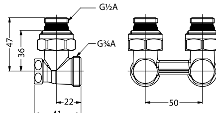
RLV-KS кутовий 003L0222
