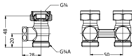
RLV-KS прямий 003L0221
